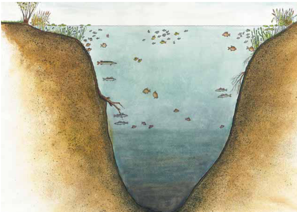
Schets van het blankvoorn-brasem diepwatertype
