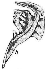
Figuur 2.1 De (linker)keeltanden van een volwassen brasem (bron: Pinder, 2001)
